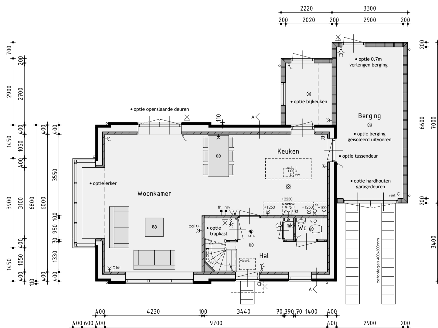
Begane grond v.z.v. vloerverwarming
